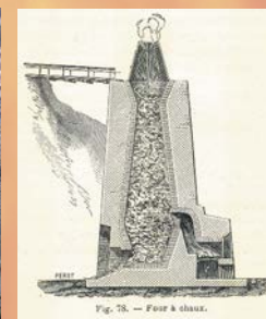
Fig. 78. — Four à chaux.
